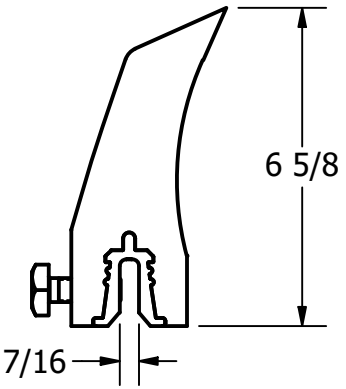
E1x Blade Profile
